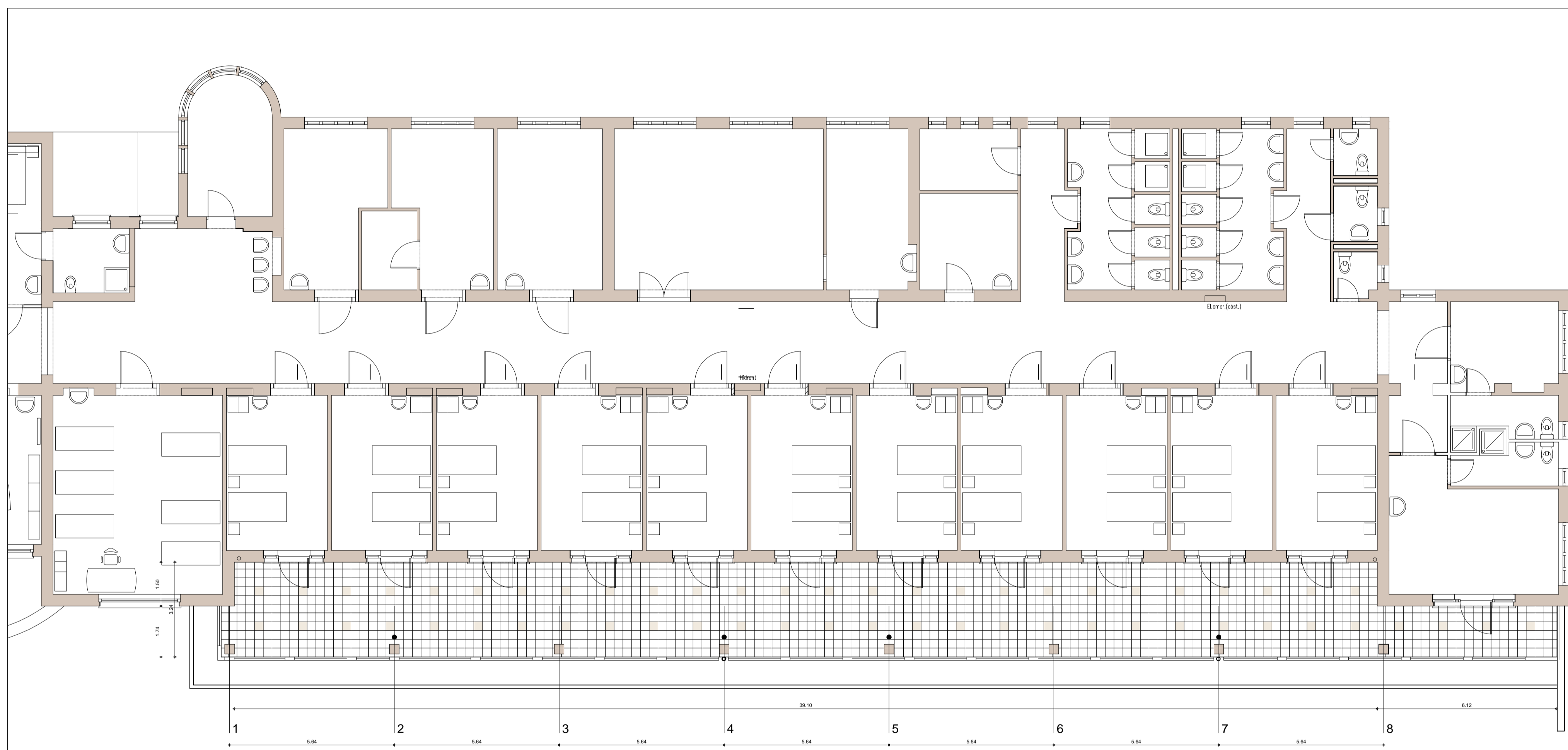
ORTOPEDSKA BOLNIŠNICA VALDOLTRA PAVILJON B SANACIJA TERAS ETAŽA B3 - SHEMA POLAGANJA KERAMIKA MERILO 1:100
